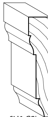
SMC-321 3/4" x 3 1/2" OG CASING
