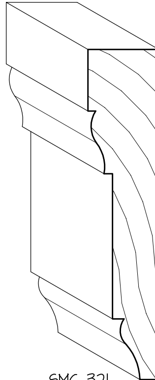
SMC-321 \frac{3}{4} " x 3\frac{1}{2} " OG CASING
